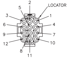
VOIR FIL A-A VUE D'INSERTION
